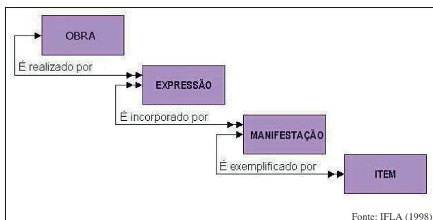
FIGURA 1 – Modelo Entidade-Relacionamento Grupo 1
