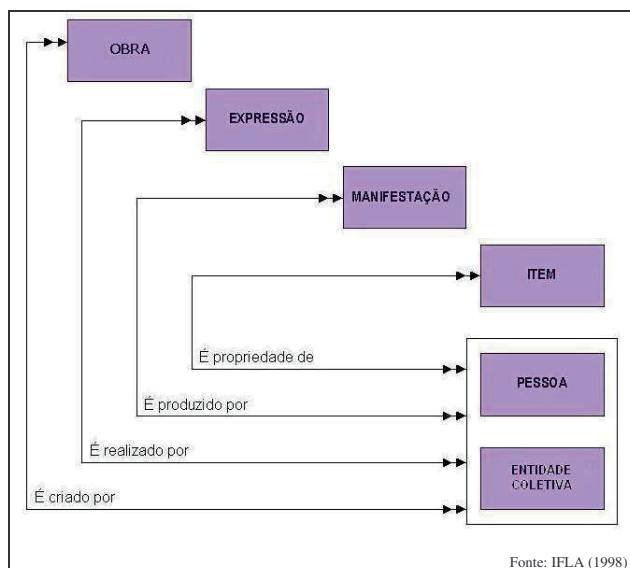
FIGURA 2 – Modelo Entidade-Relacionamento Grupo 1 e 2
