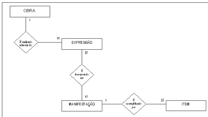
FIGURA 9 – Diagramação original do MER - Exemplo
