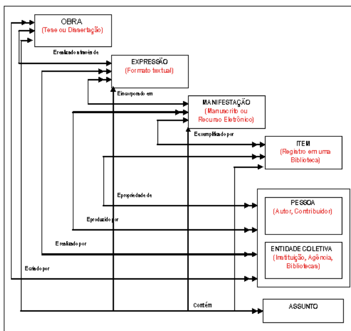
FIGURA 10 - Teses e Dissertação no Modelo FRBR
