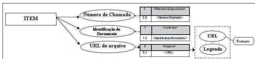
FIGURA 18 - Entidade ITEM e seus atributos
