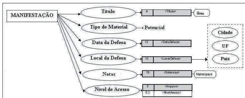
FIGURA 17 - Entidade MANIFESTAÇÃO e seus atributos
